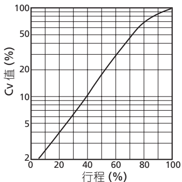
图 1 等百分比特性
