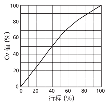
图 2 线性特性 流量特性
